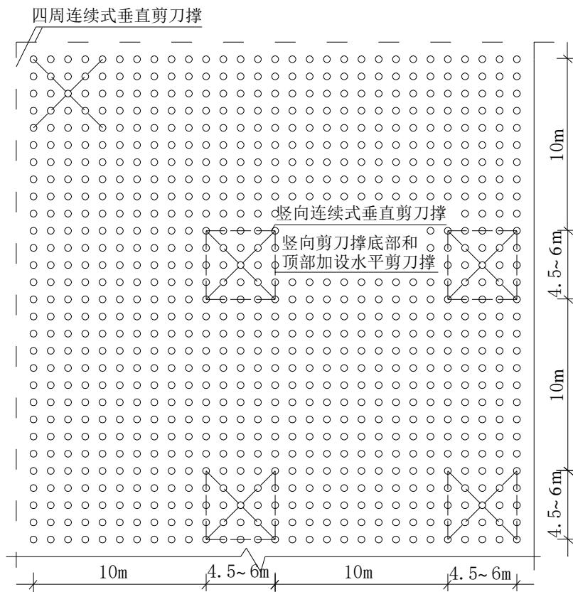
图 6.2.4-1 剪刀撑布置图（一）
