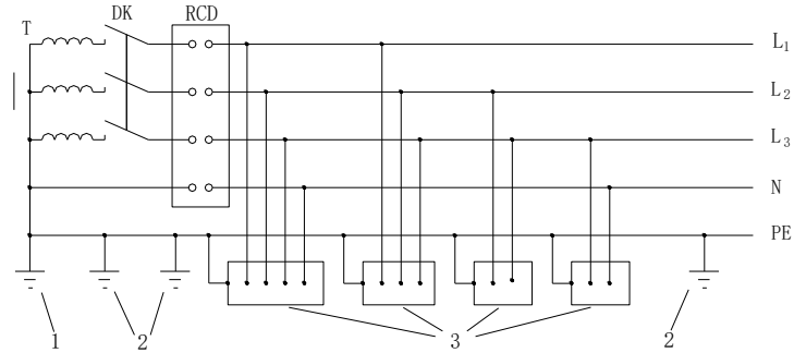
1—工作接地；2—PE 线重复接地；3—电气设备金属外壳（正常不带电的外露可导电部分）；L 1 、L 2 、L 3 —相线；N—工作零线；PE—保护零线；DK—总电源隔离开关；RCD—总漏电保护器（兼有短路、过载、漏电保护功能的漏电断路器）；T—变压器
