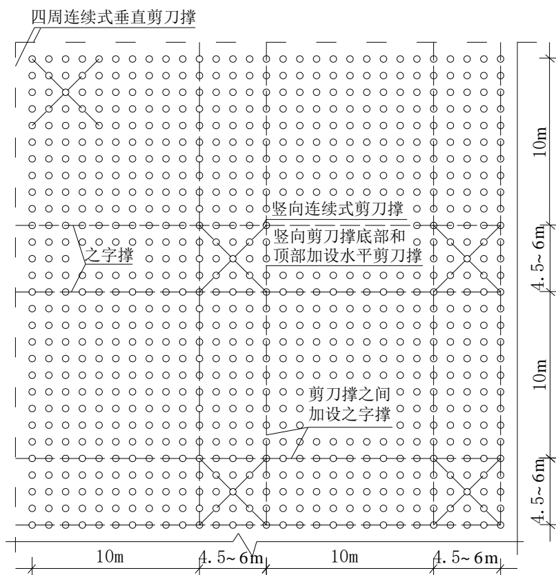
图 6.2.4-2 剪刀撑布置图 (二)
