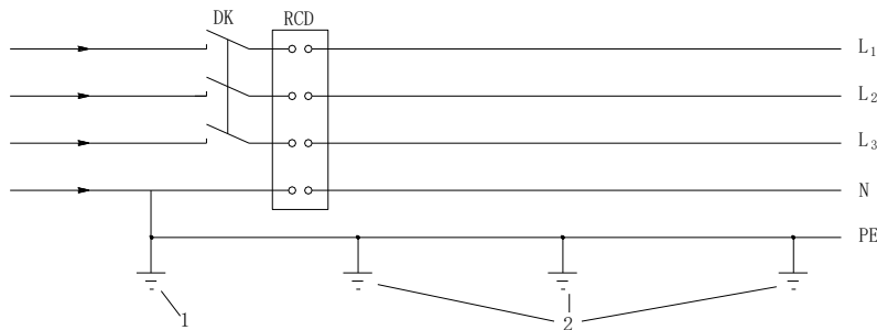
1—NPE 线重复接地；2—PE 线重复接地；L 1 、L 2 、L 3 —相线；N—工作零线；PE—保护零线；DK—总电源隔离开关；RCD—总漏电保护器（兼有短路、过载、漏电保护功能的漏电断路器）
